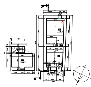
PŮDORYS 1.PP
