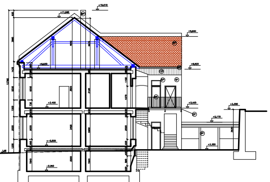
ŘEZ A-A
