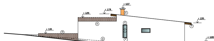
POHLED JZ
